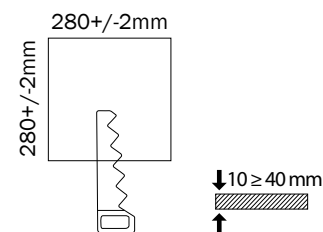
Infällningsöppning (300x300 mm)
